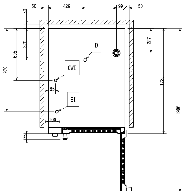
Boven aanzicht
